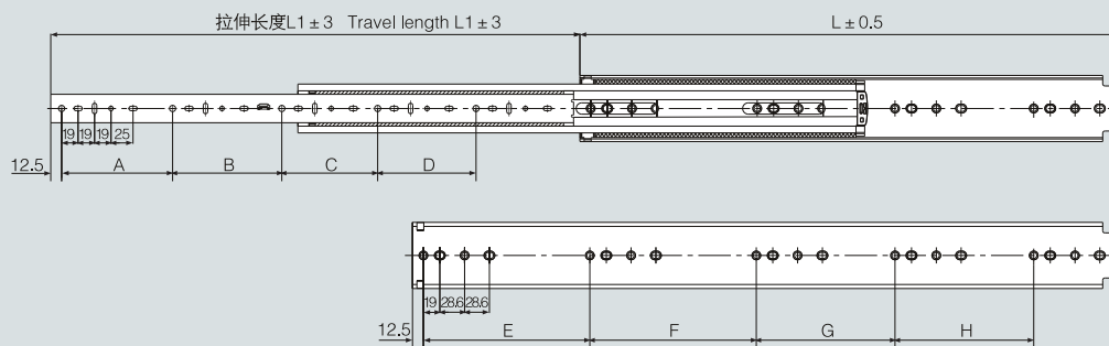
滑轨安装孔尺寸 Hole pattern
