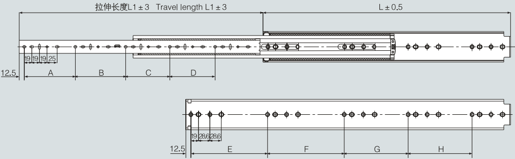
滑轨安装孔尺寸 Hole pattern
